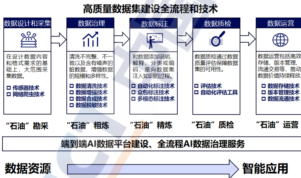
图4 高质量数据集建设全流程和技术
